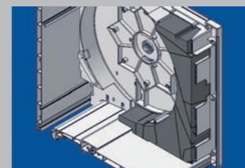
Kopfstückdämmung möglich
